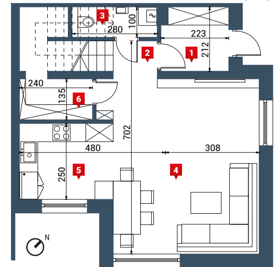
Rzut parteru
