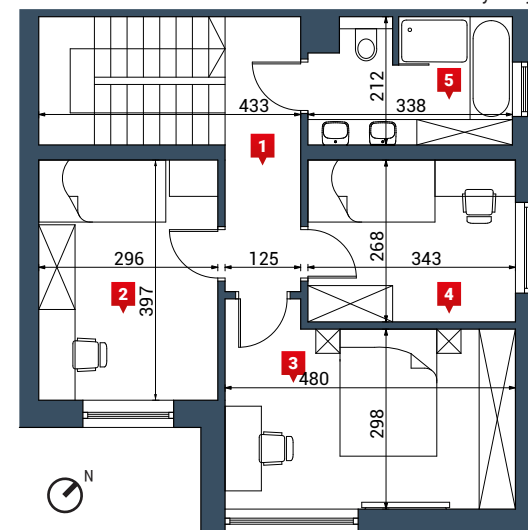
Rzut piętra
